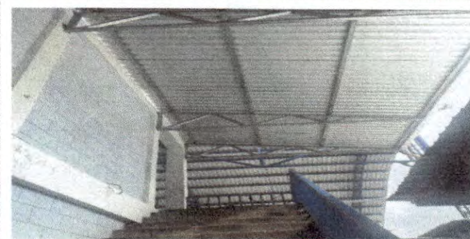
Foto 11: INSTALACION DE ESTRUCTURA, DE METAL PARA CUBRIR MODULO DE GRADAS, ACCESO AULAS SEGUNDO NIVEL.
